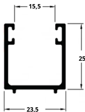
U-1108 0,345 Kg/m
