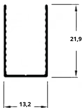
ABC-010 0,109 Kg/m
