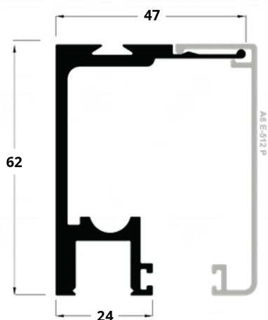
L-537 1,271 Kg/m
