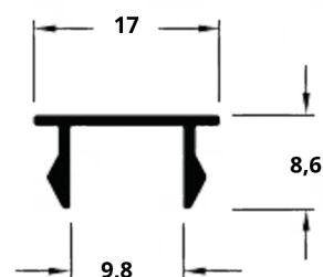
U-491 0,103 Kg/m
