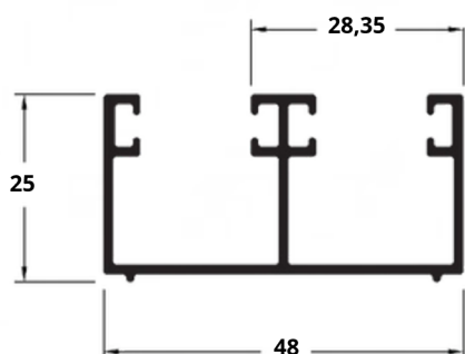
CR-247 0,552 Kg/m
