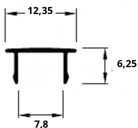
ABC-1504 0,045 Kg/m
