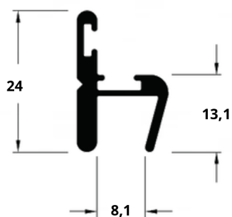
A6-343B 0,295 Kg/m
