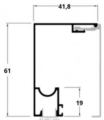
ABC-211E 0,565 Kg/m
