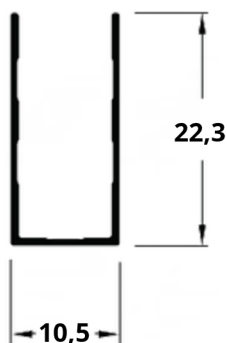
ABC-008 0,108 Kg/m
