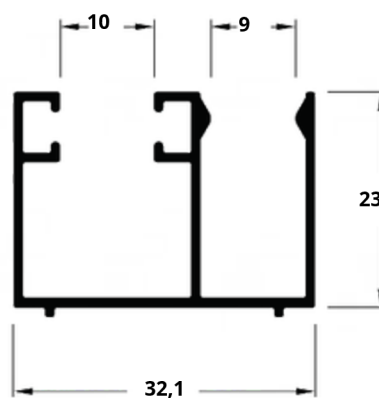
CM-173 0,425 Kg/m
