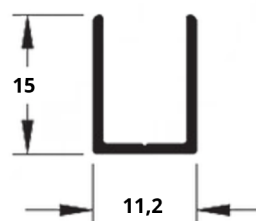
CRA-932 0,122 Kg/m
