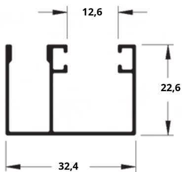
CRA-9641 0,293 Kg/m
