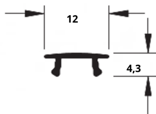
AL-027 0,045 Kg/m
