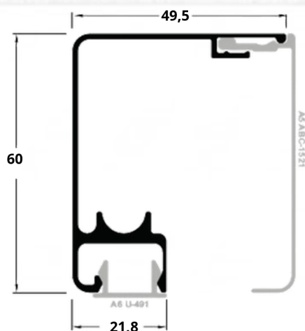
ABC-1520 0,682 Kg/m
