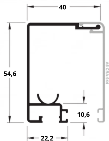
CRA-943 0,557 Kg/m
