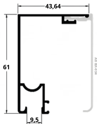
BX-036 0,587 Kg/m
