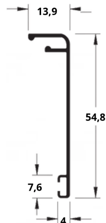
CRA-944 0,213 Kg/m
