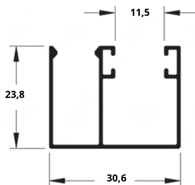
AL-003 0,265 Kg/m
