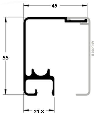
L-573B 0,694 Kg/m
