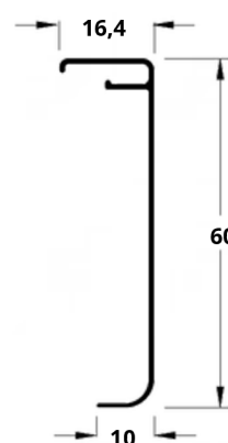
AL-052 0,241 Kg/m
