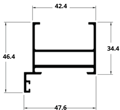
A6 42-012 0,813 kg/m
