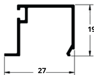
U-1076 0,192 kg/m
