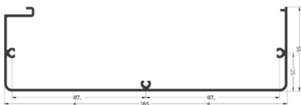
MI-114 1,422 Kg/m
