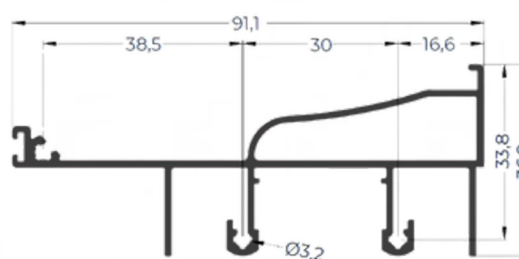
PRM20-I02 0,951 Kg/m
