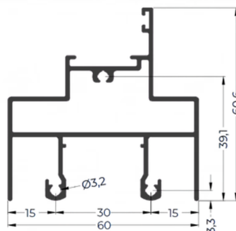
PRM20-M41 1,081 Kg/m
