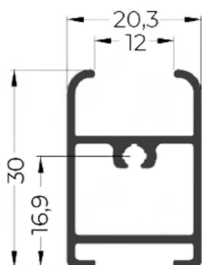
PRM20-M22 0,377 Kg/m
