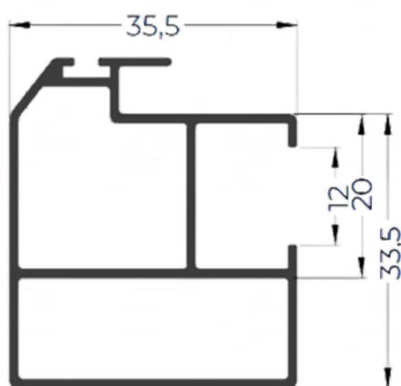
PRM20-F07 0,579 Kg/m
