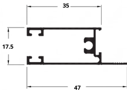
MP-309 0,382 Kg/m
