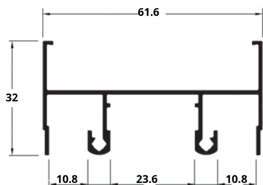
ALU-125 0,626 Kg/m
