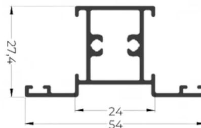
PRM20-M25 0,551 Kg/m
