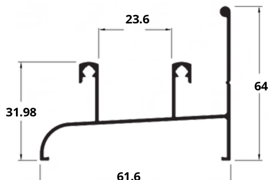
ALU-126 0,613 Kg/m
