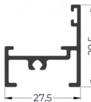
PRM20-M24 0,340 Kg/m
