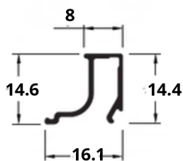
ALU-030 0,117 Kg/m
