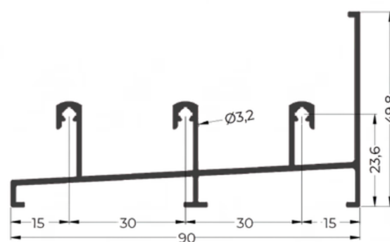
PRM20-M04 0,886 Kg/m
