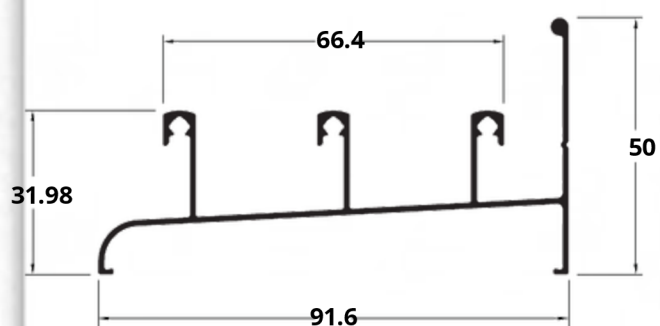
ALU-030 0,117 Kg/m
