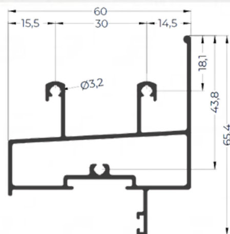
PRM20-M39 0,996 Kg/m
