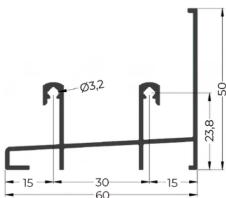
PRM20-M1 0,670 Kg/m
