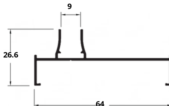
ALU-127 0,401 Kg/m
