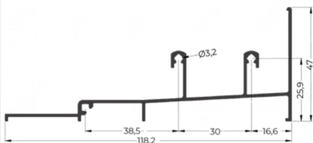
PRM20-IO1 0,817 Kg/m Trilho inf. int. 2 Planos (M)
