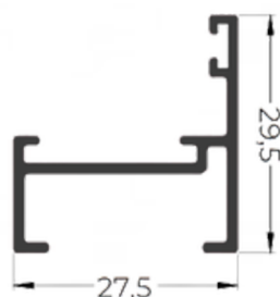
PRM20M24SO 0,303 Kg/m
