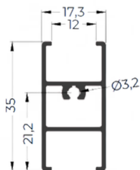
PRM20-F10 0,352 Kg/m
