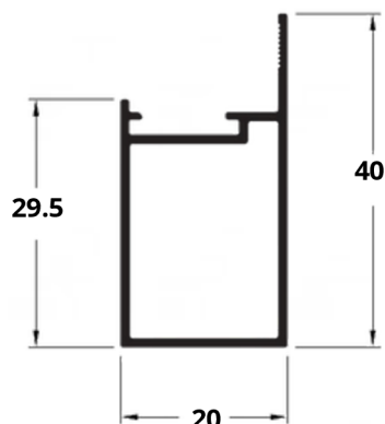
MP-300 0,324 Kg/m
