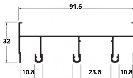
ALU-135 0,857 kg/m
