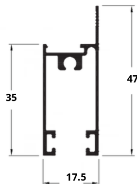
MP-309 0,382 Kg/m
