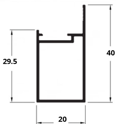
MP-300 0,324 kg/m
