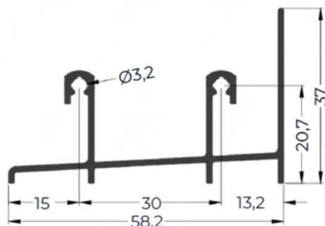
PRM20-M12 0,543 Kg/m
