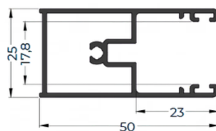
MI-322 0,604 Kg/m
