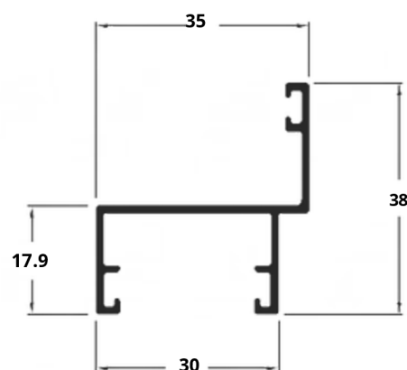
A6 Y-140 0,384 Kg/m
