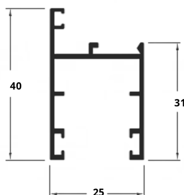
A6 Y-195 0,445 kg/m
