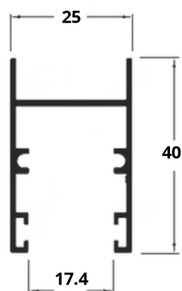
A5 I-122 0,465 kg/m
