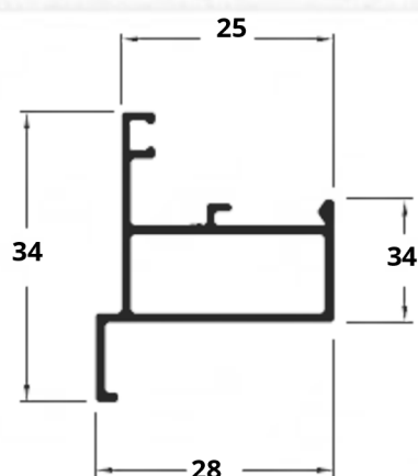
A5 P-167 0,350 kg/m
