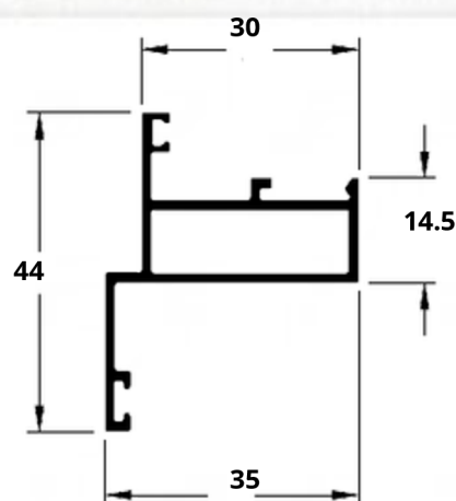
A6 P-120 0,508 kg/m
