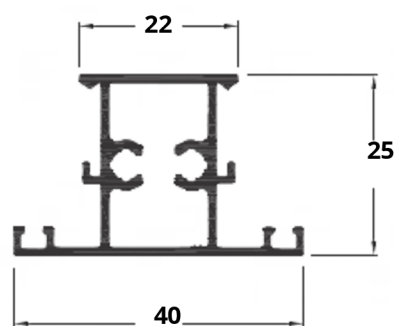
A5 P-153 0,494 kg/m
