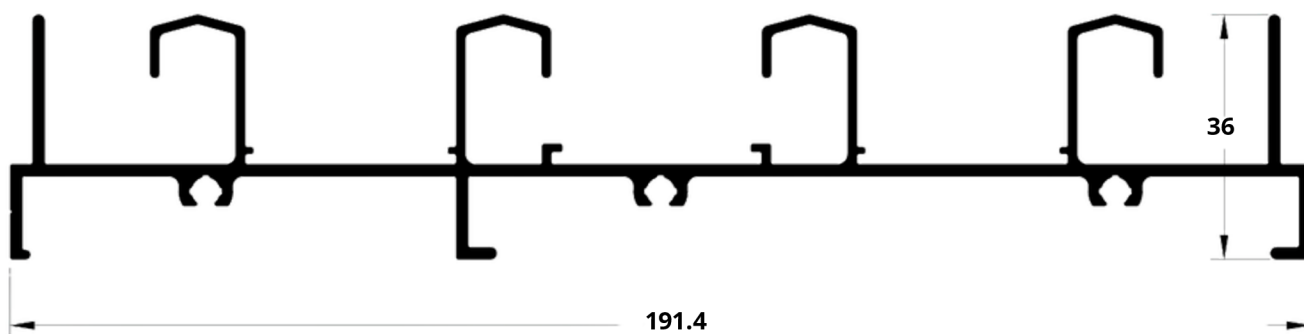
A6 LG-070 2,176 kg/m TRILHO SUPERIOR 4 FOLHA
