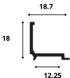
A5 LG-015 0,142 kg/m
