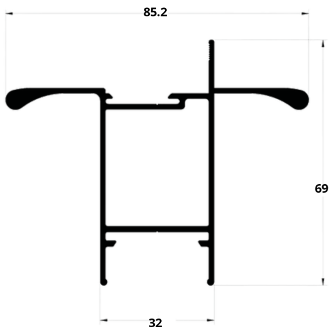
A6 LG-201 1,202 Kg/m
