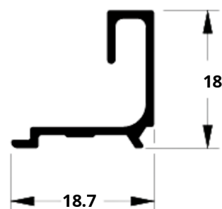
A6 LG-027 0,147 kg/m
