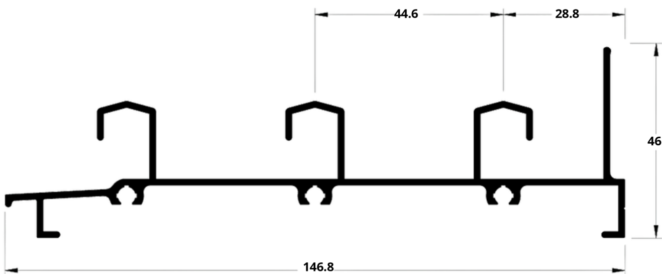
A6 LG-066 1,417 kg/m TRILHO INFERIOR 3 FOLHA
