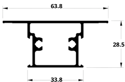
A6 LG-055 0,706 kg/m
