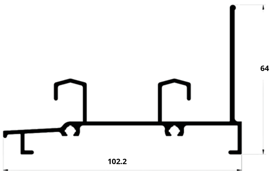
A6 LG-024 1,264 kg/m
