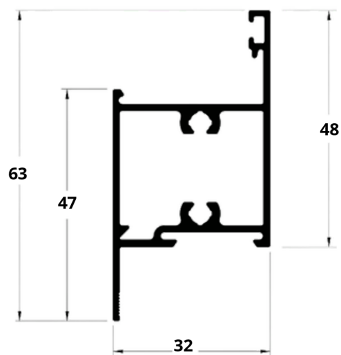
A5 LG-076 0,766 kg/m
