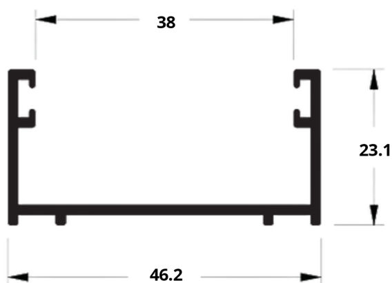
A6 LG-028 0,455 kg/m
