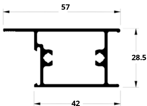
A6 LG-058 0,747 kg/m
