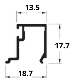
A4 BG-057 0,167 kg/m BAGUETE
