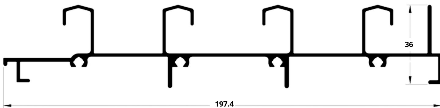
A6 LG-071 1,250 Kg/m
