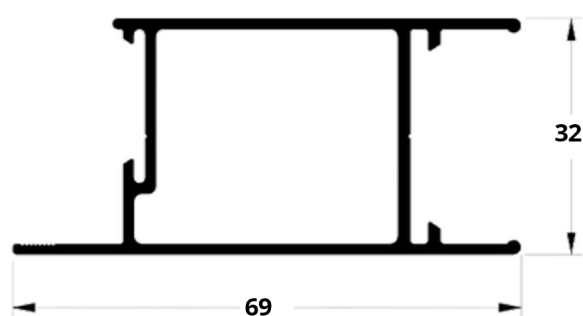
A6 LG-050 0,729 kg/m
