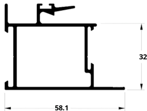
A6 LG-049 0,815 Kg/m
