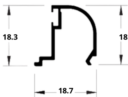
A6 LG-026 0,159 kg/m
