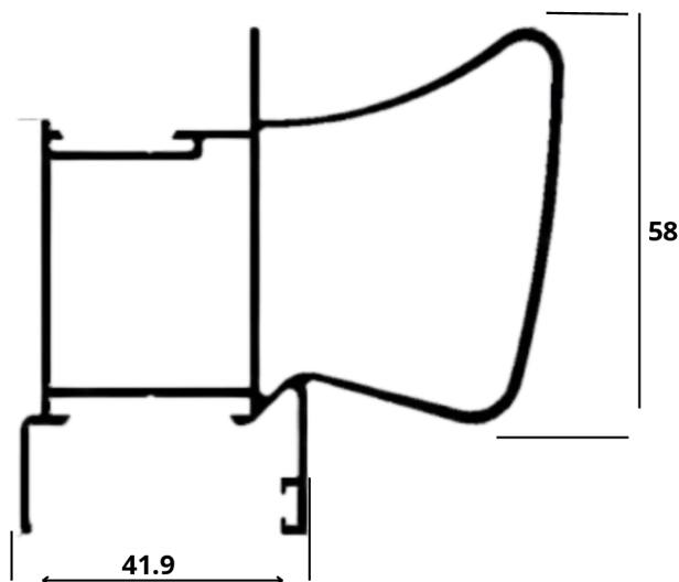
A5 LG-139 1,624 kg/m
