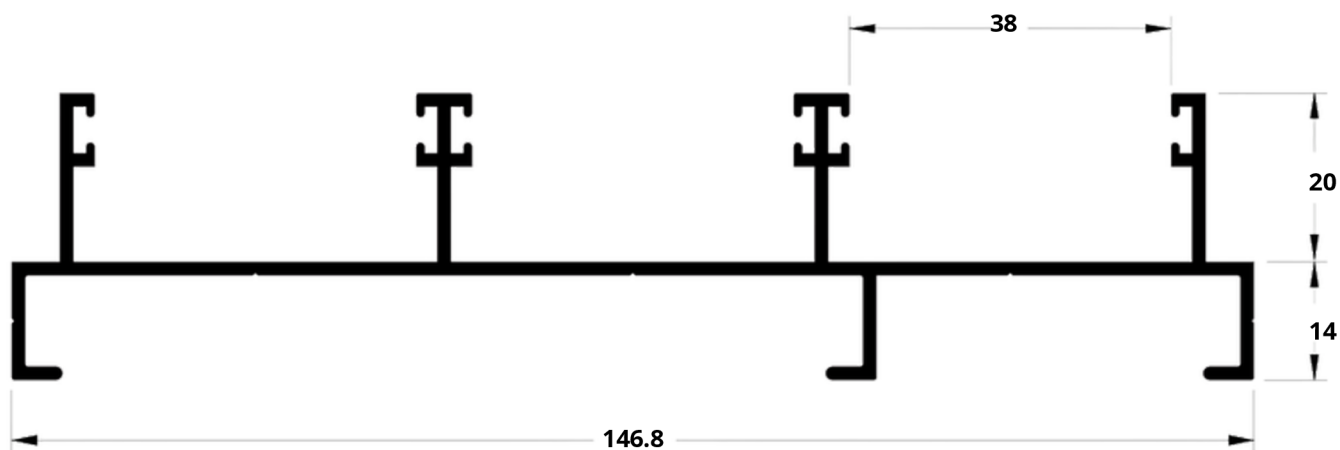
A6 LG-064 1,250 Kg/m MARCO LATERAL 3 FOLHAS
