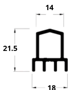
A6 LG-061 0,319 Kg/m TRILHO AVULSO - LINHA GOLD
