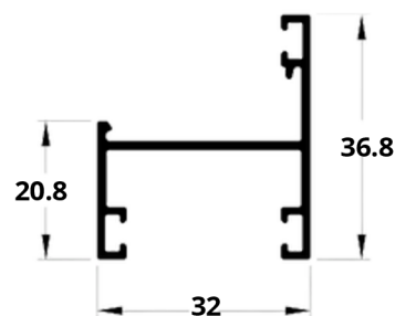
A6 LG-068 0,369 kg/m MARCO MAXIM AR
