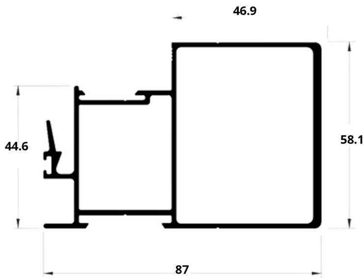
A6 LG-052 1,581 kg/m
