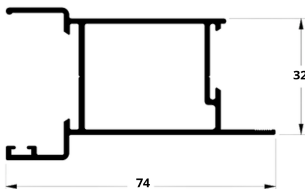
A6 LG-051 0,831 kg/m
