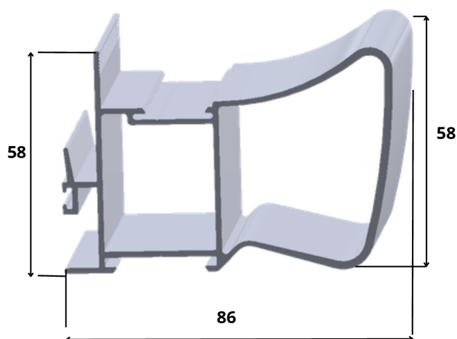
A6 LG-137 1,578 kg/m
