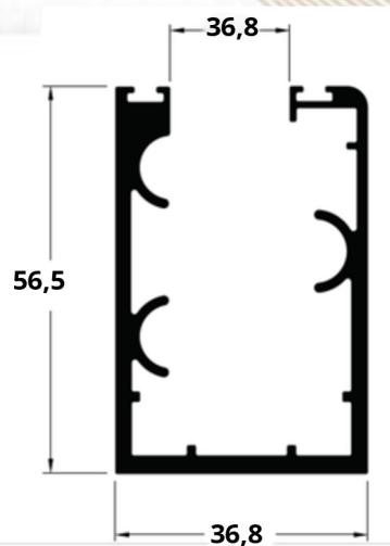
A6 AE-158 1,256 Kg/m
