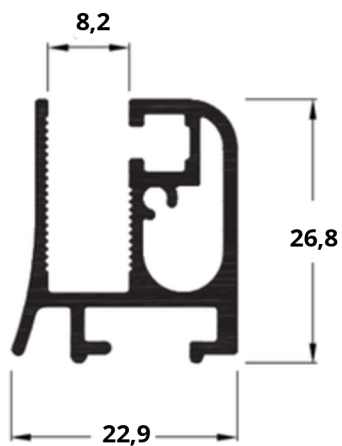
A6 AE-160 0,467 Kg/m
