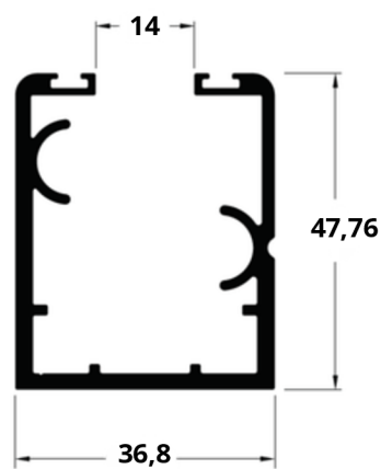
A6 AE-157 0,983 kg/m
