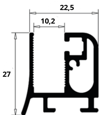
A6 AE-159 0,473 Kg/m
