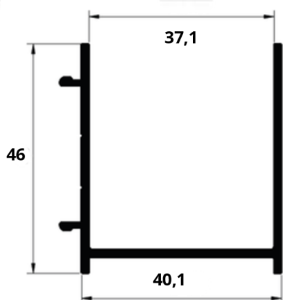
A6 AE-156 0,561 kg/m
