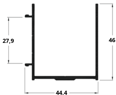
A6 AE-156A 0,591 Kg/m
